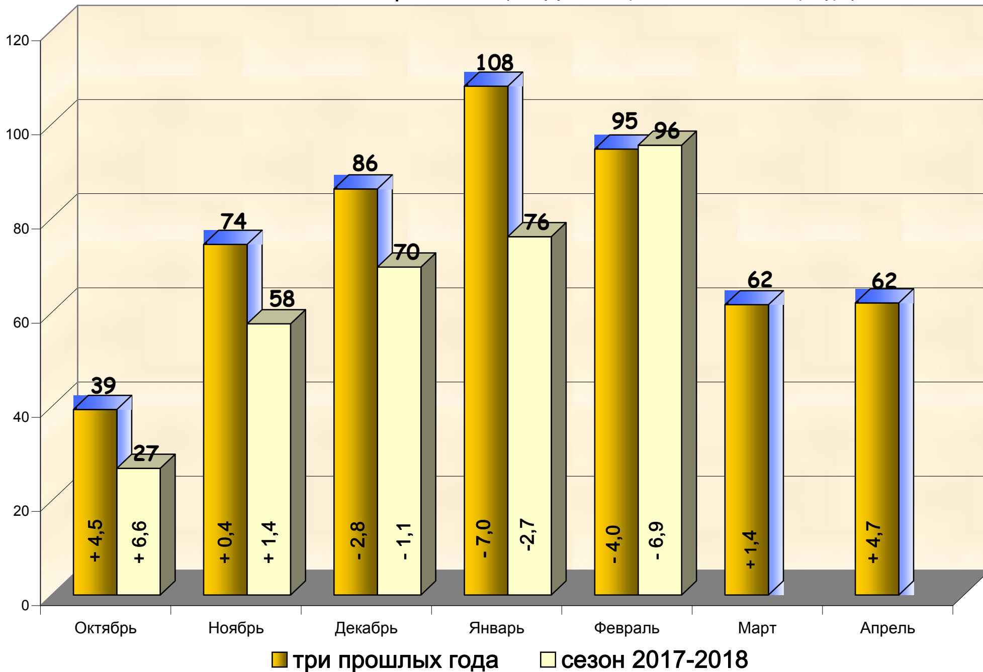
Сколько затрачено тепла на отопление, Гкал. Сравнение текущего отопительного сезона с прошлыми. (внизу указана среднемесячная температура)
