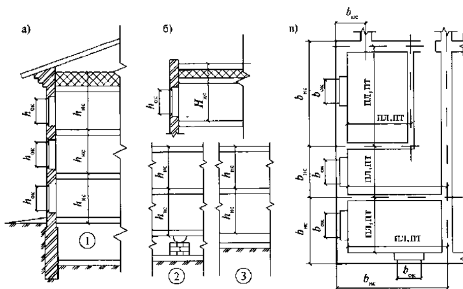
Рисунок 1 – Правила обмера площадей ограждающих конструкций: а – разрез здания с чердачным перекрытием; б – разрез здания с совмещенным покрытием; в – план здания; 1 – пол над неотапливаемым подвалом; 2 – пол на лагах; 3 – пол на грунте
