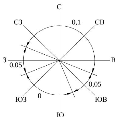
Рисунок 3 – Величины добавок к основным теплопотерям в зависимости от ориентации наружной ограждающей конструкции по сторонам света
